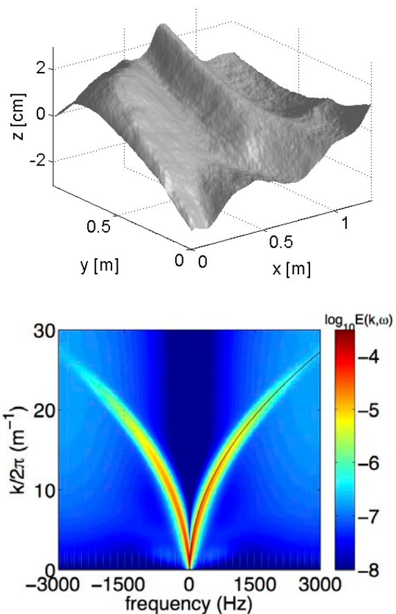
En haut: exemple de déformation d'une tôle vibrée en acier, mesurée à 10000 images/s. En bas: spectre spatiotemporel des ondes de flexion sur une telle plaque montrant un spectre turbulent d'ondes faiblement non linéaire. On observe des fréquences allant du Hz à plusieurs kHz.
